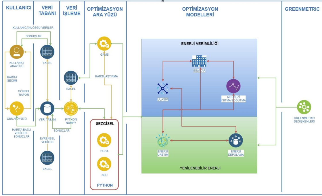
Şekil 1 - Kampüs Enerji Planlama ve Optimizasyon Modeli Bileşenleri
